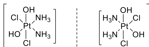
enantiomers
