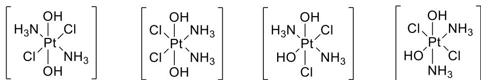
oxaplatin
