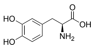
L-DOPA
