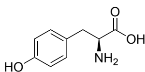
L-Tyrosine
